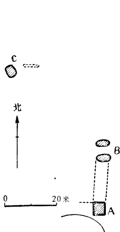
图5 K778平面图
