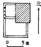
圖 21 T128 (烏蘭松治) 平面图
