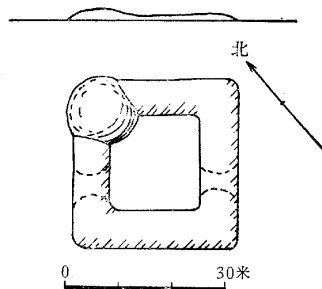
圖 32 F159平、剖面圖
