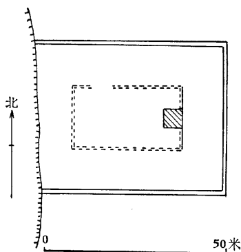
图29 T148平面图
