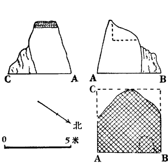
圖 26 K823 平、剖面圖
