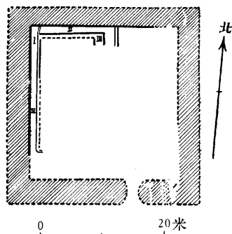
圖1 A1(宗間阿瑪)平面圖
