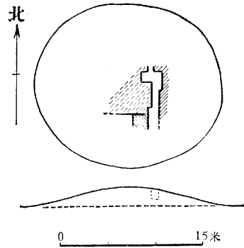
图9 A14平、剖面图
