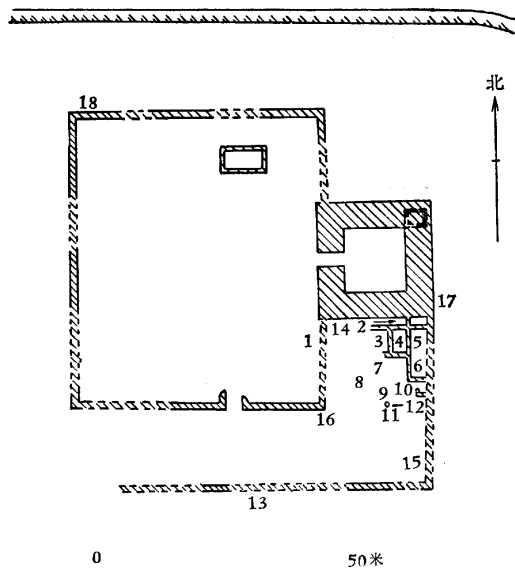
图34 A33(地湾)平面图
