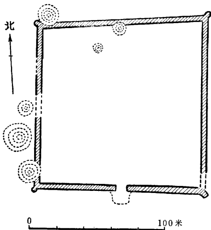
圖7 K710(居延城)平面圖
