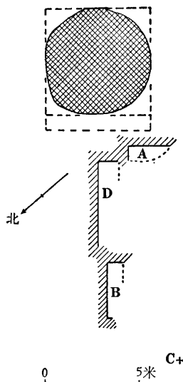
图30 A27(查科尔帖)平面图
