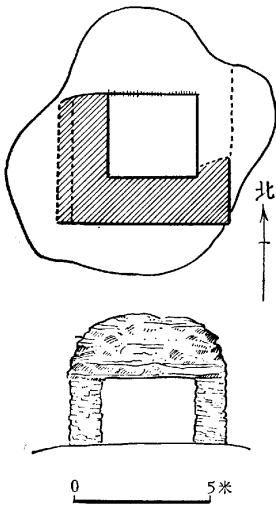
圖2 A10(瓦因托尼)平面及正視
