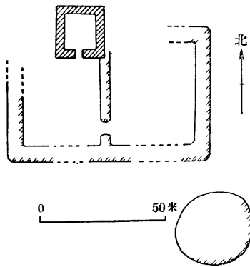
圖 27 A24 (小方城) 平面圖
