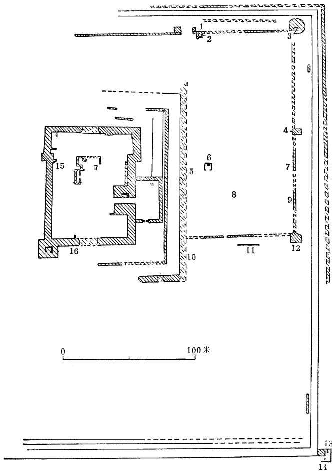
圖 36 A35 (斯氏 T48d 大灣城) 平面圖
