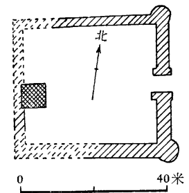
圖 28 K822 (大方城) 平面圖
