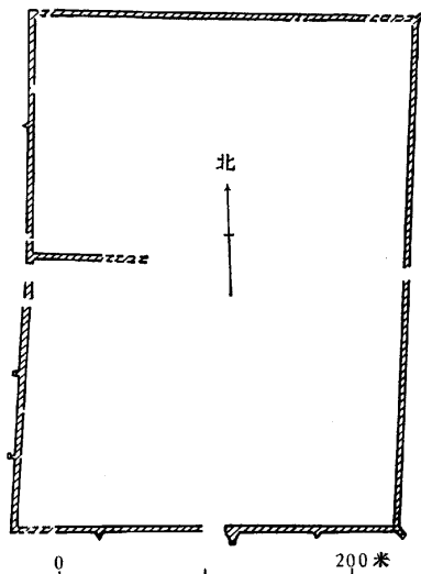
圖 38 A38 (斯氏 T47 蒙漢城) 平面圖
